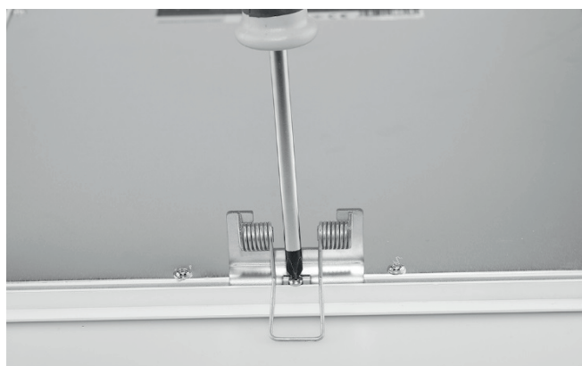
Abb. 7: Federbügel für LED Panel Gemma
