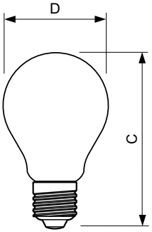
filament 7W-60W 808lm NAD 2700K E27D
