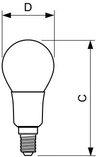
filament 2.5W-25W 250lm NAD 2700K E14D
