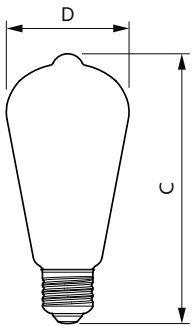
ST64 230V 60W 806lm 2700-2200K E27 D CL
